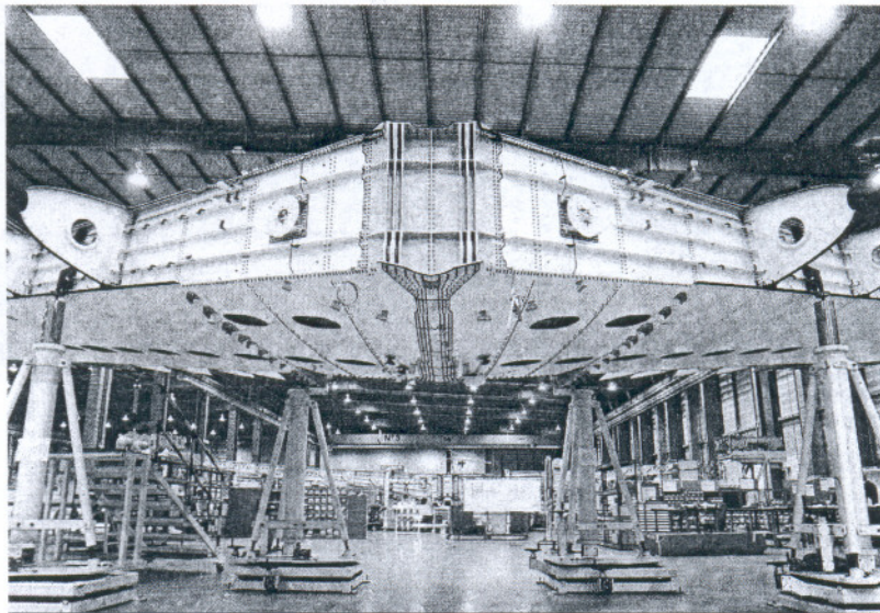
Interior de la factoría de Airbus Puerto Real, en los trabajos de construcción del A380.
